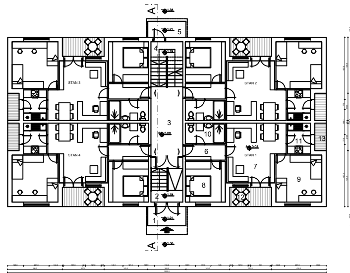
OSNOVA PRIZEMLJA R=1:100
