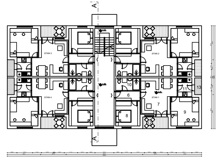
OSNOVA SPRATA R=1:100
